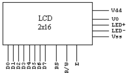
Gambar 7. Modul LCD
