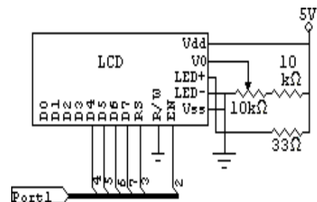
Gambar 13. Rangkaian LCD
