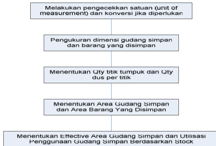
Gambar 3. Metodologi penentuan effective area gudang simpan dan utilisasinya
